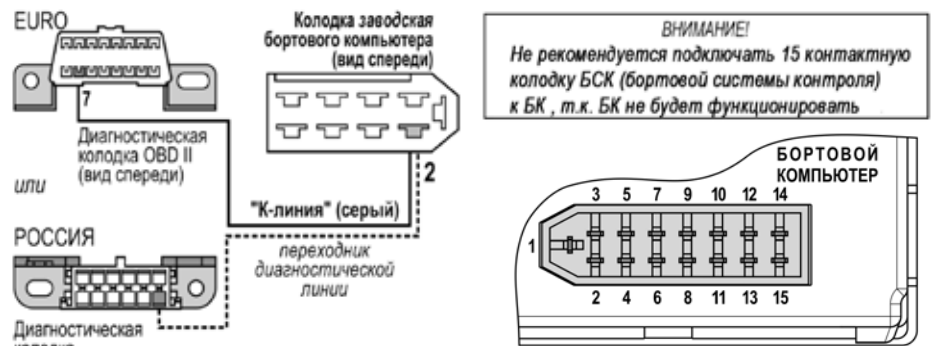
Рис.1 Схема подключения (обычная панель) схема контактов БК
