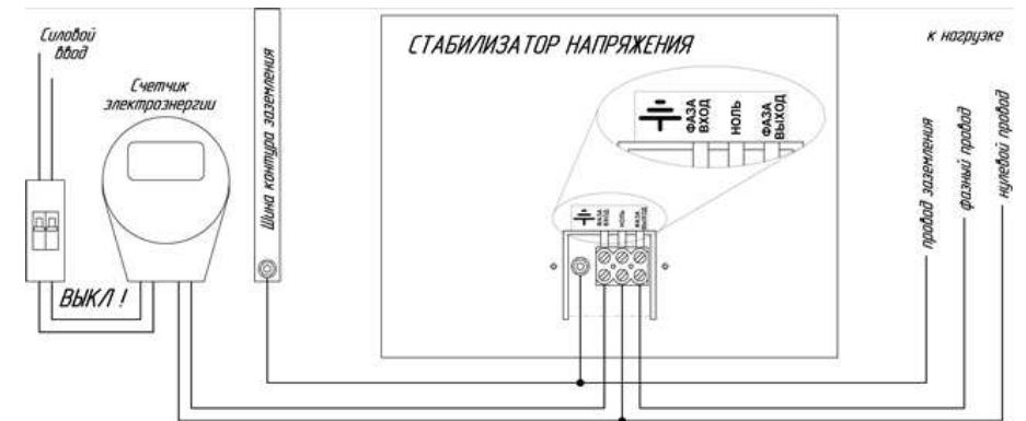
Рисунок 2. Рекомендуемая схема подключения стабилизатора к сети.
