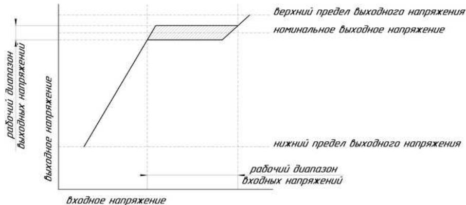
Рисунок 1. Передаточная характеристика стабилизатора напряжения.
